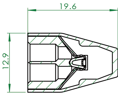
剖面 B-B
